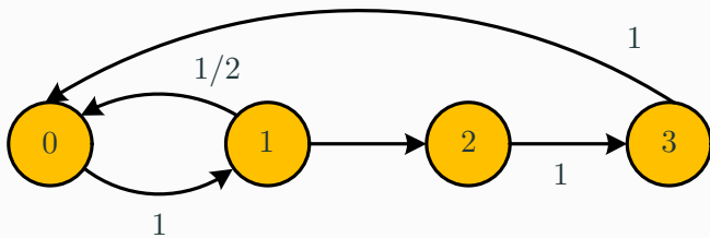
Figura 2: Uma classe - cadeia irredutível.
