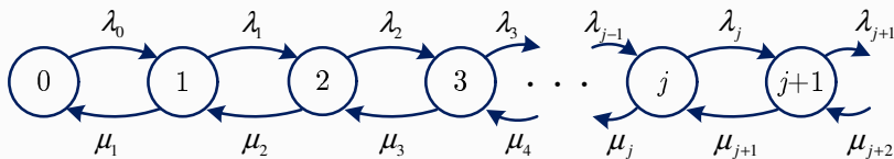
Figura 4: Diagrama de transição de um processo de nascimento-e-morte.
