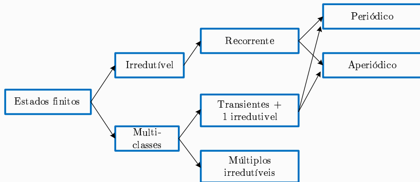
Figura 3: Possíveis estruturas para cadeias de Markov.
