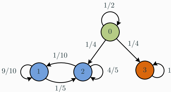
Figura 1: Três classes: \{0\} , \{1, 2\} e \{3\} .
